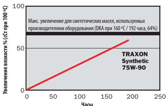
Испытание на окисляемость ДКА (СЕС-Л-48-А-95) (192 часа при 160 °С) GL-5 75W-90 Synthetic
