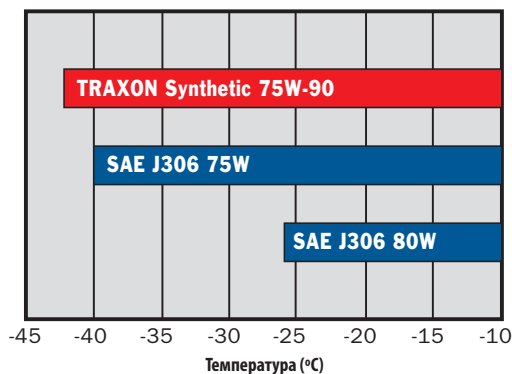
Сравнение температуры, при которой вязкость масла TRAXON и GL-5 (°C) составляет 150 000 сП
